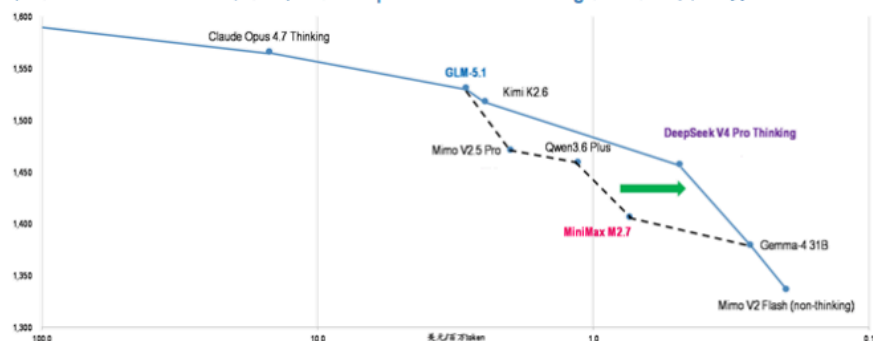
图 2：Arena WebDev 帕累托前沿：DeepSeek V4-Pro Thinking 重设低成本优势
